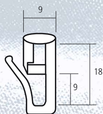
Gleiter 2403
