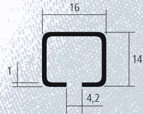
u4-Alu-Schiene, Profil
