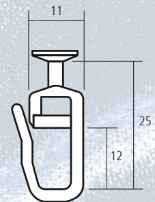
Gleiter 2430
