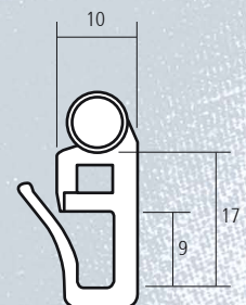
Laufroller 2421
