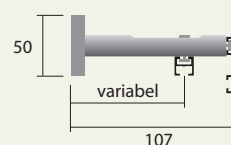
2-läufig Art. 871 2281:
