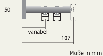
2-/3-läufig Art. 871 2281:
