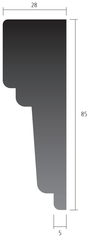
Blendenhöhe 8,5 cm
